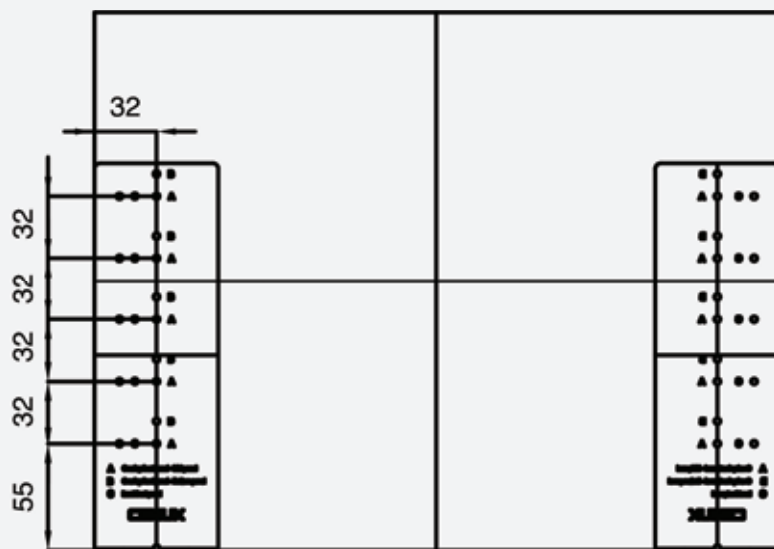
H Box & A Box čelní příchyt (Středový panel) - Otvor A
