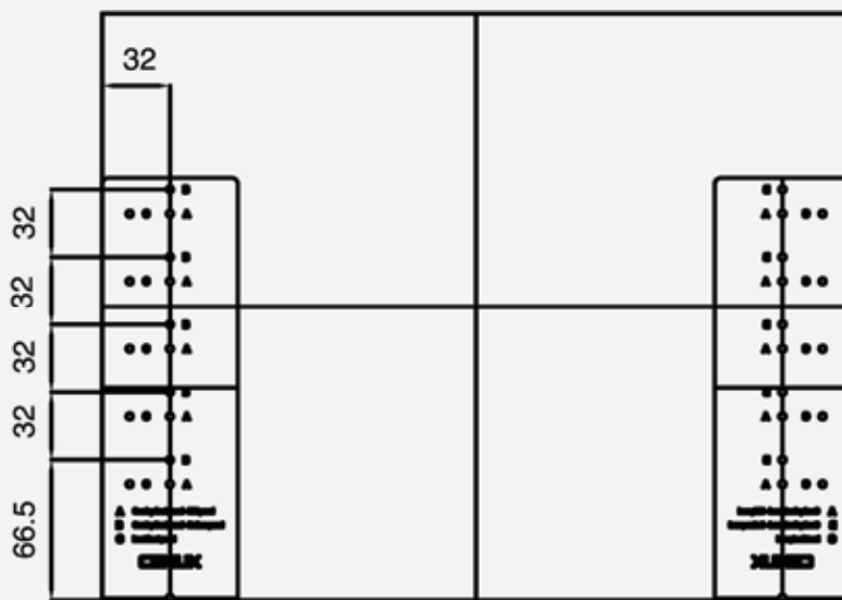
H Box & A Box čelní příchyt (Spodní panel) - Otvor B
