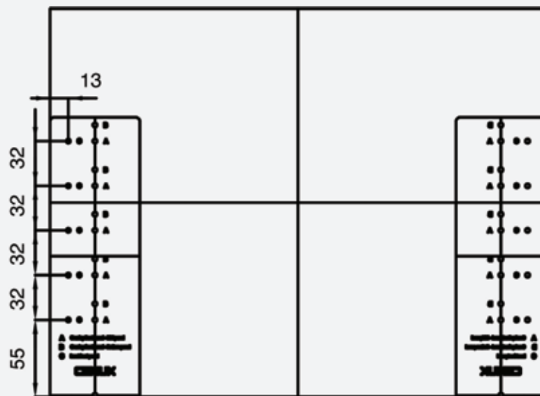
H Box & A Box čelní přichyt - Otvor C
